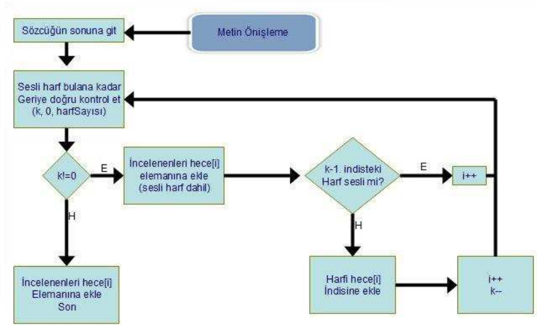
Şekil 2.8 : Heceme algoritması akış diyagramı
